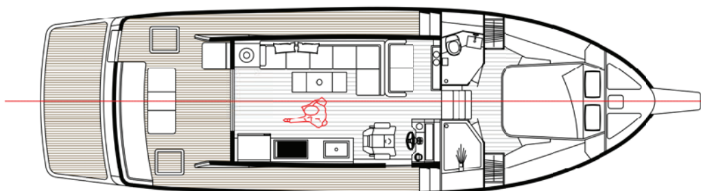
GENERALE ARRANGEMENT
