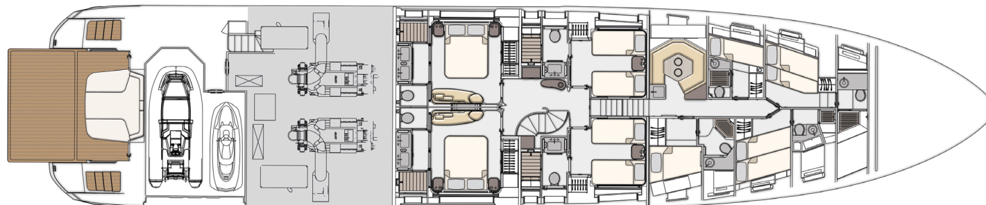
LOWERDECK
