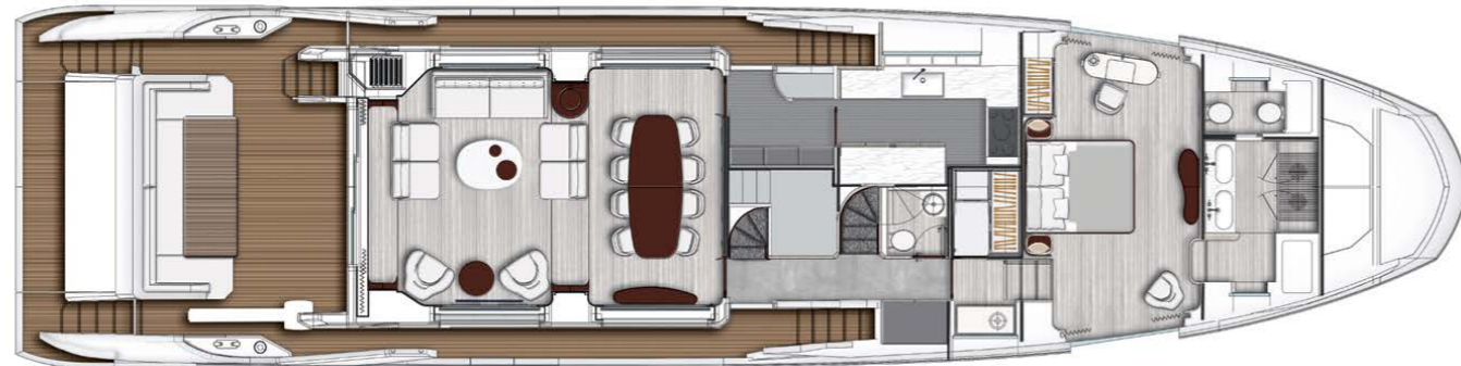
Maindeck
