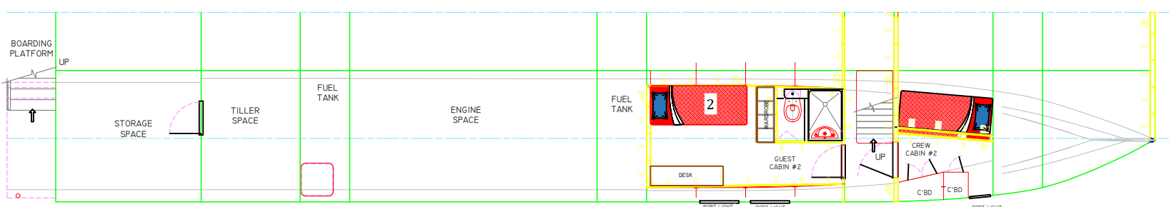
4 HULL DECK SCALE: 1:50
